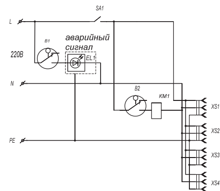
Принципиальная схема ТОПАС 100
